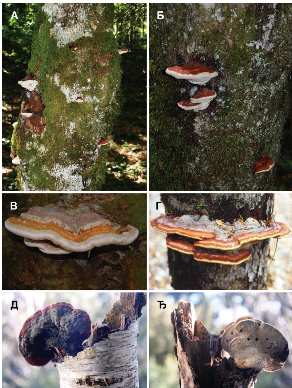
Слика 4. Fomitopsis pinicola – плодоносна тела на: А-Б-В – букви ( Fagus sylvatica L.), Г – сивој јови ( Alnus incana (L.) Moench), Д-Љ – брезе ( Betula pendula Roth.)
