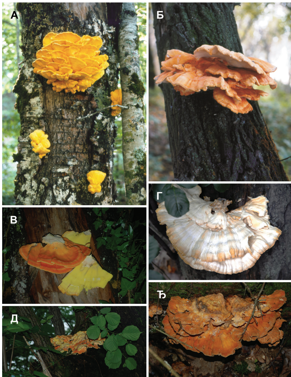
Слика 5. Laetiporus sulphureus - плодносна тела на: А - стабљу букве ( Fagus sylvatica L.), Б - врби ( Salix sp.), В - дивљој трешњи ( Prunus avium L.), Г - црном јасену ( Fraxinus ornus L.), Д - црној јови ( Alnus glutinosa (L.) Gaertn.), Ђ - китњаку ( Quercus petraea (Matt.) Lieblein)
