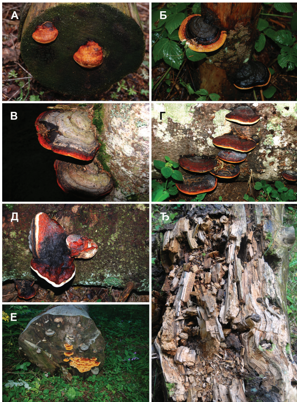
Слика 2. Fomitopsis pinicola : А-Б-В-Г- плодоносна тела на лежавинама јеле, Д. геотропизам, Ѕ - мрка призматична трулеж, Е - Fomitopsis pinicola + Gloeophyllum odoratum на истом трупцу
