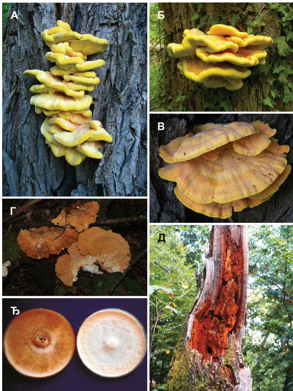
Слика 6. Laetiporus sulphureus : А-Б-В - плодоносна тела на врби, Г - на китњаку; Д - мрка призматична трулеж у стаблу китњака, Е - чиста културе гљива на хранљивој МЕА подлози (лево Fomes fomentarius , десно Laetiporus sulphureus )
